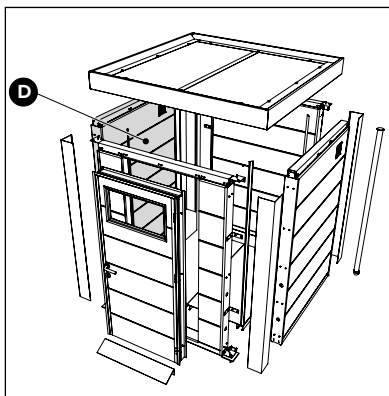
D Paroi / Wand / Wall / Wand
